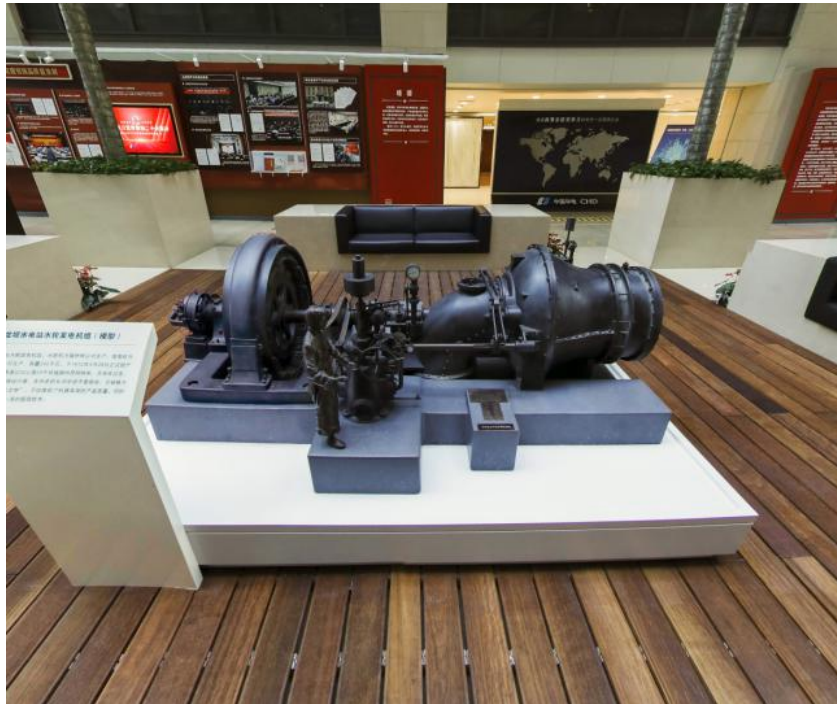
图 4 石龙坝水电站百年机组模型
